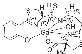
Complejo de Ga (II)-piscibactina
